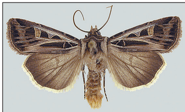
13. Dingy cutworm adult.
